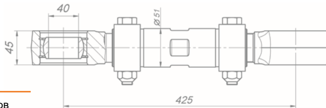
Штанга регулируемая 634-2919010
