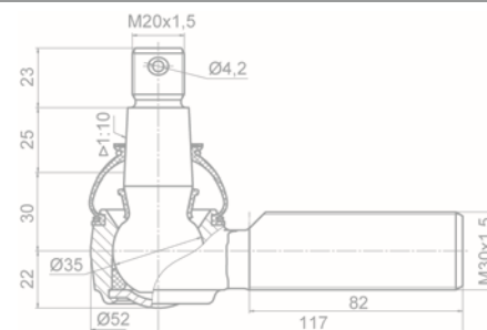
Наконечник рулевой тяги R350-3414060-20 (правый)
