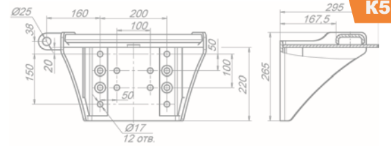
Кронштейн пневморессоры подвески верхний R65659-3011050 (правый) R65659-3011051 (левый)
