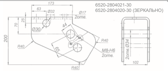
Кронштейн опорный 6520-2804020-30 (правый) 6520-2804021-30 (левый)
