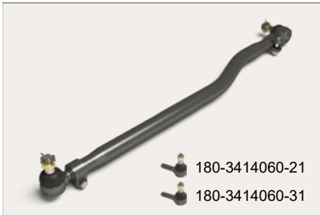
Тяга рулевая продольная правая 4525-3414010-10
