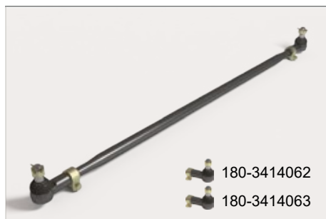
Тяга рулевой трапеции R6520-3414052
