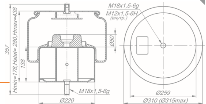
Рессора пневматической подвески 180-2934003-33
