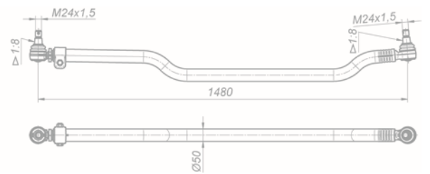
Тяга рулевой трапеции 5350-3414052
