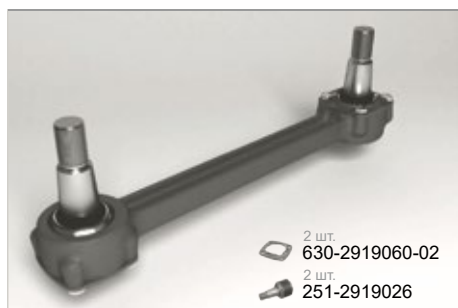
Штанга реактивная 251-2919012
