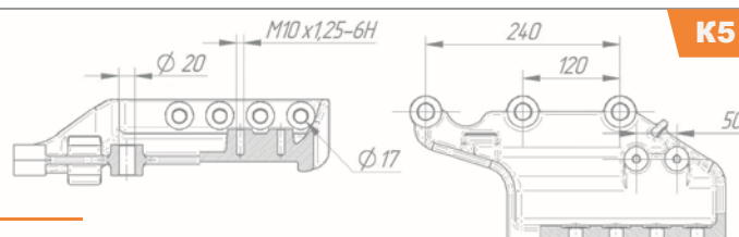
Кронштейн задний 6595-1203041-10
