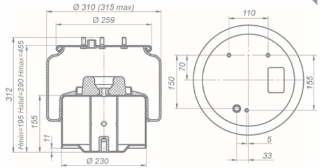
Рессора пневматической подвески 180-2934002-35
