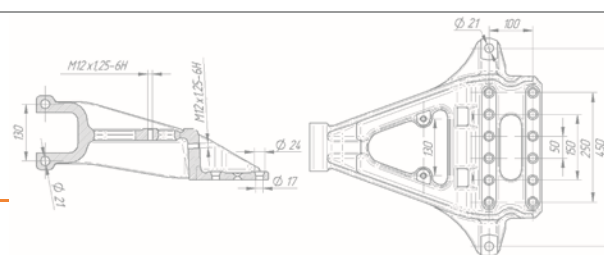
Кронштейн задней подвески 65206-2912445-47
