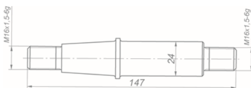
Палец крепления амортизатора P53212-2905418
