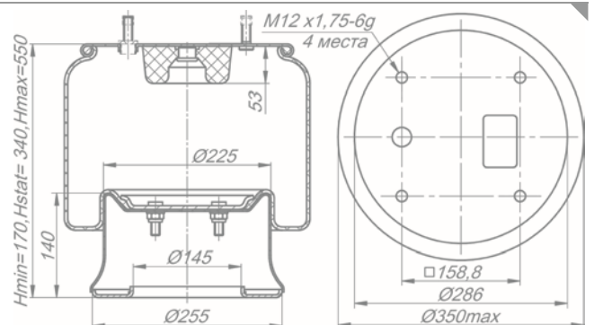
Рессора пневматической подвески 180-2934002-99
