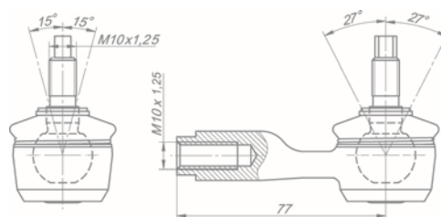
Наконечник 362-1703521-20 (правый) 362-1703522-20 (левый)
