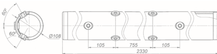
Буфер задний 6522-2804010
