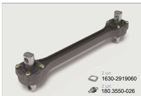
Штанга реактивная 1630-2919012-31
