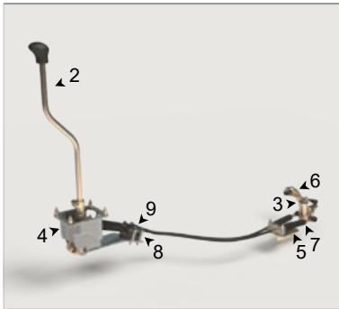
Привод управления КПП 16302-1703000
