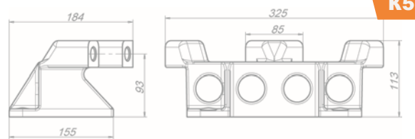
Кронштейн реактивной штанги верхней задней R65659-3011190
