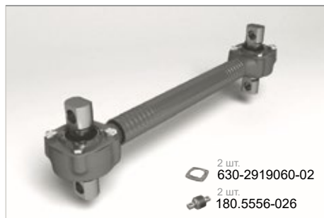
Штанга реактивная 1634-2919010
