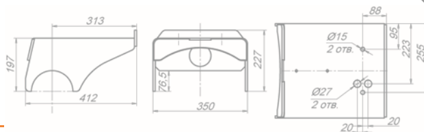
Кронштейн пневморессоры подъема оси
