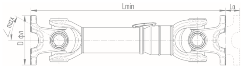
Карданные валы TD17
