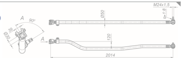
Тяга промежуточная 65801-3414130-20
