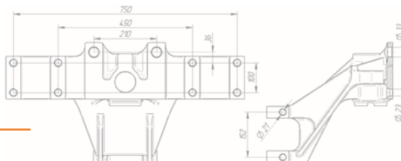
Кронштейн оси балансира 65956-2918056
