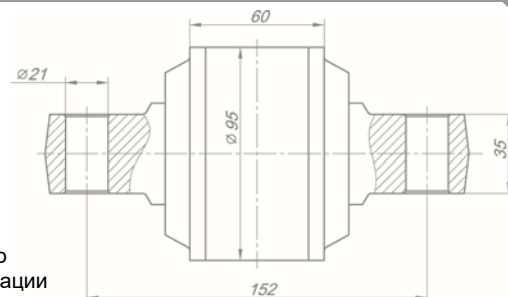
Резинометаллический шарнир 5460-2919026-40
