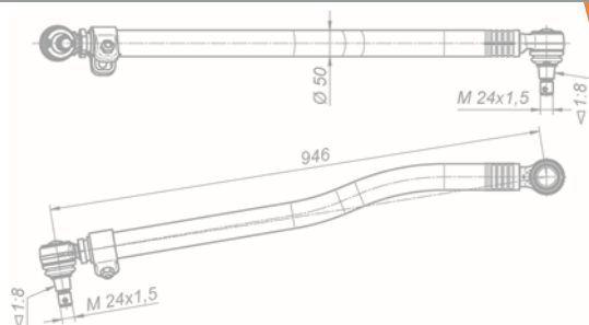
Тяга сошки 65952-3414010-20
