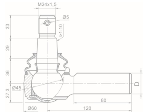
Наконечник рулевой тяги R180-3414060-20 (правый) R180-3414060-30 (левый)
