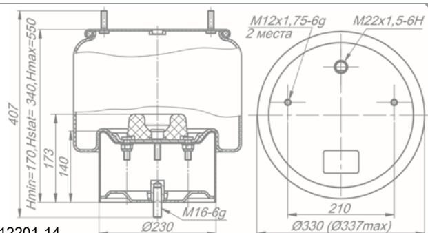
Рессора пневматической подвески 180-2934004
