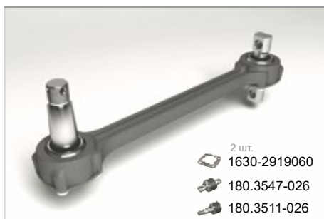
Штанга реактивная 1630-2919012-10 1630-2919012-11 1630-2919012-12
