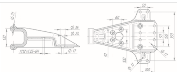
Кронштейн задней подвески 5490-2912445-45
