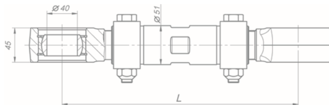
Штанга реактивная 634-2919010-11 634-2919010-23 634-2919010-24 634-2919010-25 634-2919010-26
