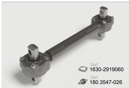
Штанга реактивная 1630-2919010-50
