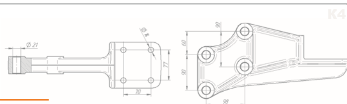
Кронштейн нижний 5490-2809050-10
