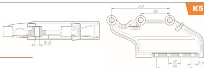
Кронштейн задний 65951-1203041
