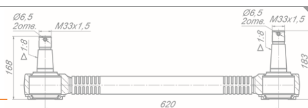
Штанга реактивная верхняя 620-2919010-10Э
