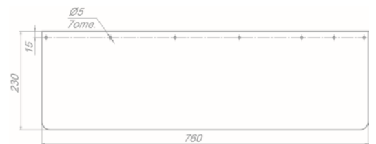
Брызговик облицовочной панели 43114-8401450-04
