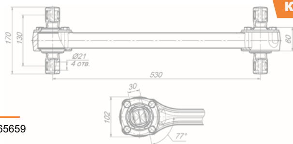
Штанга реактивная 1630-2919012-31
