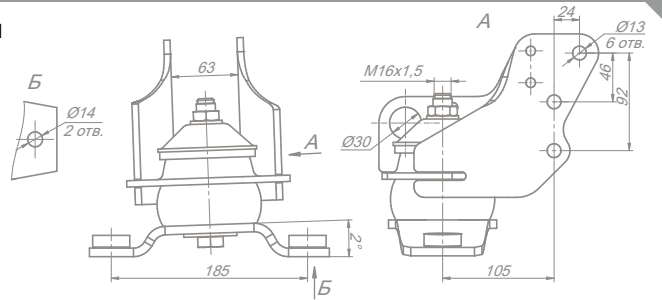
Опора передняя правая 650.1001019-20
