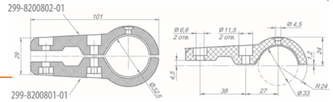
Кронштейн перегородки 299-8200800-01
