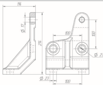
Вставка лонжерона R6580-2918158 (правая) R6580-2918159 (левая)
