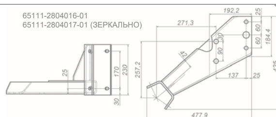
Кронштейн буфера 65111-2804016-01 (правый) 65111-2804017-01 (левый)
