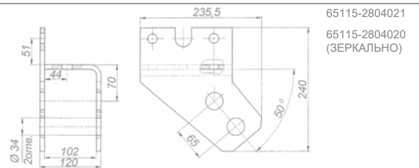
Кронштейн опорный 65115-2804020 (правый) 65115-2804021 (левый)
