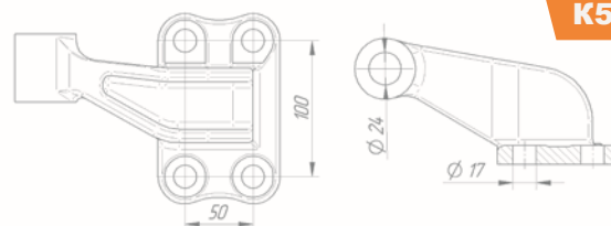
Кронштейн амортизатора верхний 65951-2905510 (правый) 65951-2905511 (левый)
