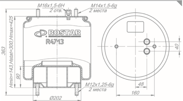
Рессора пневматической подвески 180-2934003-23
