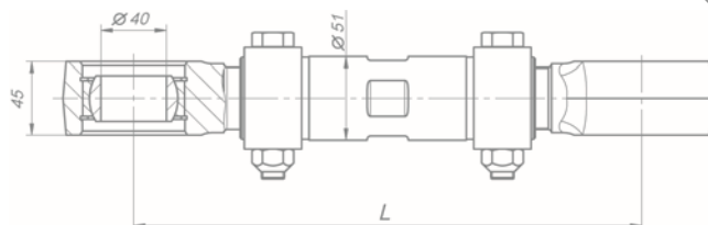
Штанга реактивная 634-2919010-10 634-2919010-20 634-2919010-21 634-2919010-22
