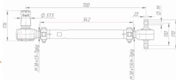
Штанга задней подвески верхняя 529265-2919014-03
