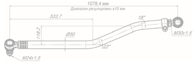
Тяга рулевая продольная 180-3414010-481
