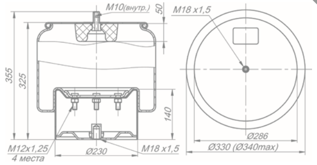
Рессора пневматической подвески 180-2934002-03
