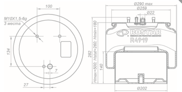
Рессора пневматической подвески 180-2934002-105
