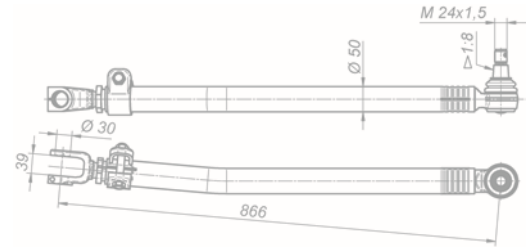
Тяга сошки с наконечниками 65225-3414010-11
