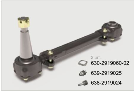
Штанга задней подвески нижняя 529265-2919016-23
