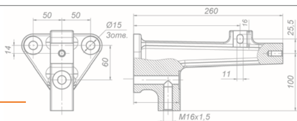
Кронштейн передней опоры кабины 65956-5001035-10
