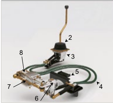
Комплект тросового привода переключения КПП 530-1703000
