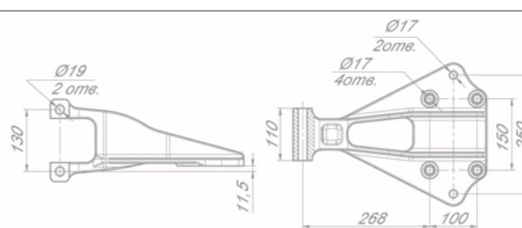
Кронштейн задней подвески R43083-2912445
