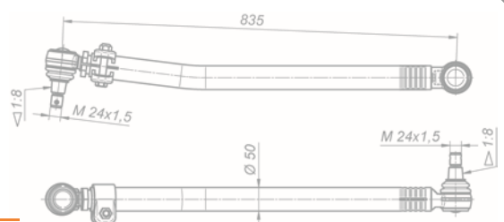
Тяга сошки с наконечниками 6520-3414010-41
