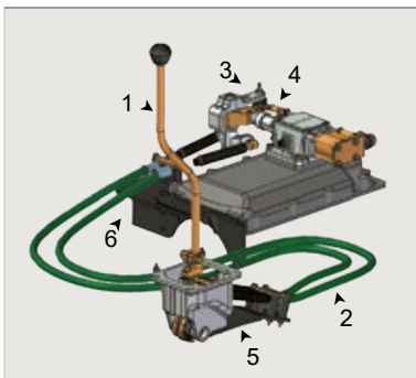
Привод управления КПП 536-1703003
