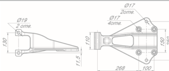
Кронштейн задней подвески
