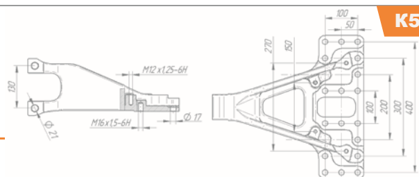
Кронштейн задней подвески 54901-2912447-10
