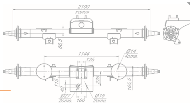
Балка оси R65208-3011500-03
