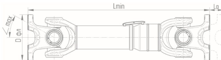
Карданные валы TS17
