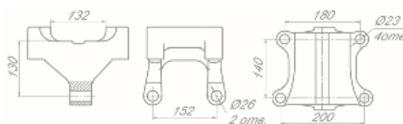
Рычаг нижний задний правый R65117-2919182
